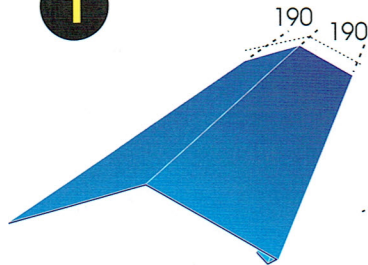
Gąsior płaski
