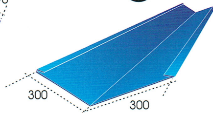
Rynna koszowa
