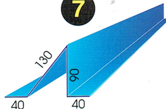
Bariera śniegowa
