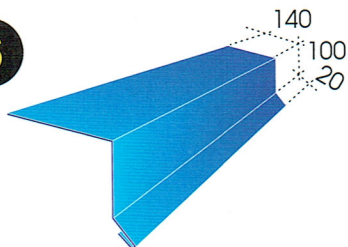
Obróbka wiatrownicy
