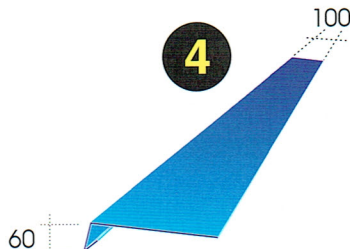
Pas nadrynnowy
