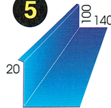
Obróbka komina
